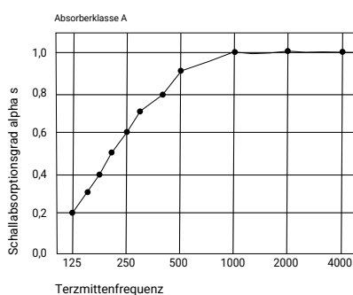
SCHALLSAUGER® Frameless Montage ohne Deckenabstand
