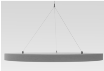
Montage mit 3:1 Drahtseilabhängung und Bohrschablone. Mindestabstand zur Decke 34 cm.
