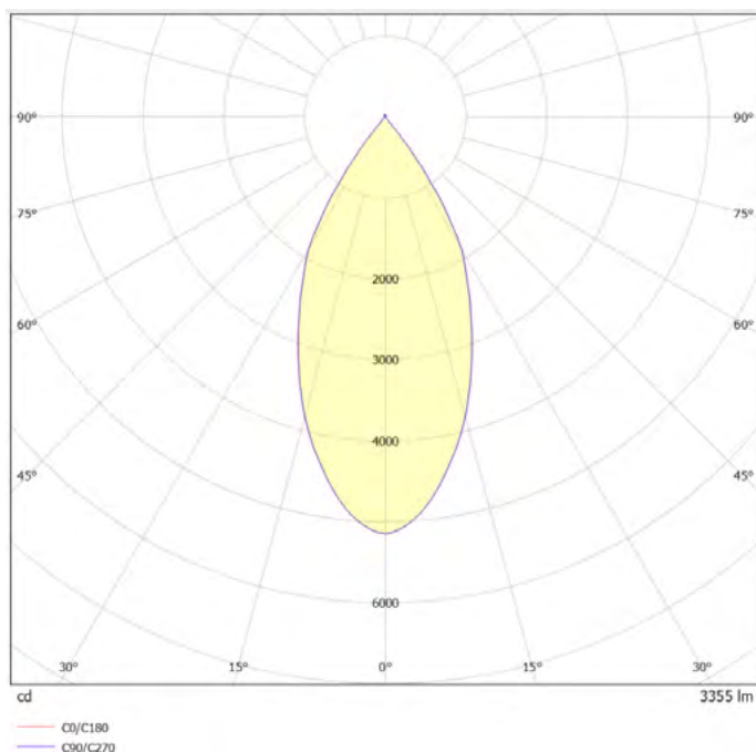
Lichtstärkeverteilungskurve
