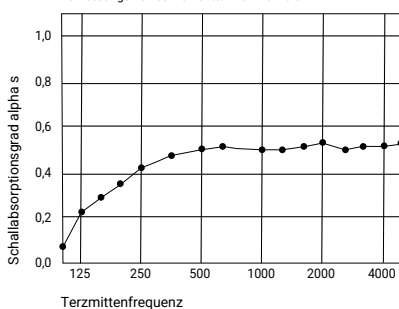
SCHALLSAUGER® Frameless Baffle Abstand zwischen den Elementen 60 cm
