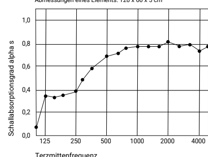
SCHALLSAUGER® Frameless Baffle Abstand zwischen den Elementen 60 cm
